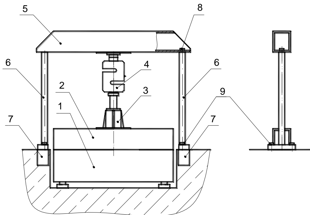
1 – Блок роликов; 2 –Балка опорная; 3 – Силозадающее устройство (домкрат); 4 – Динамометр; 5 – Балка верхняя; 6 – Стойка; 7 – Закладной брусок; 8 – Болт, 9 – Болт.
