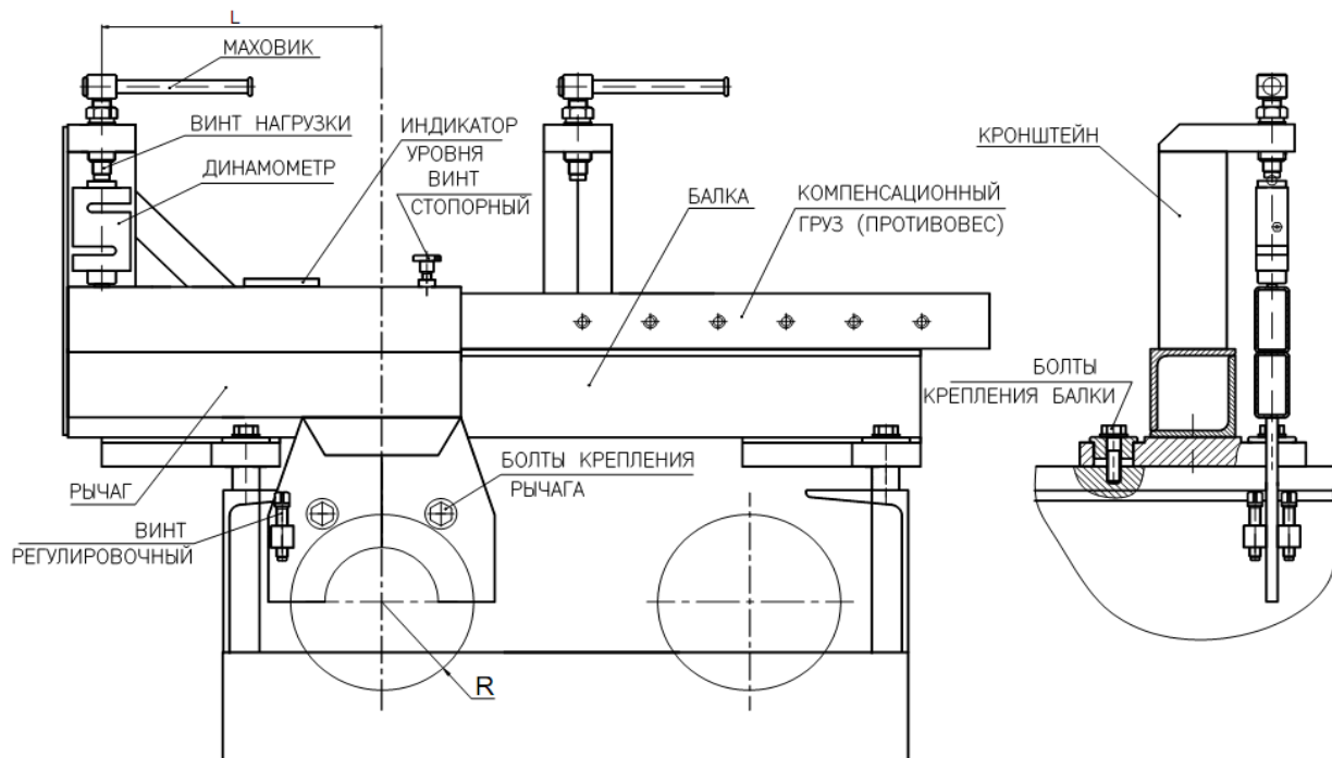
Рис.7 Рычаг поворочный для поверки датчиков тормозной силы тормозного стенда СТН 3000М.01
