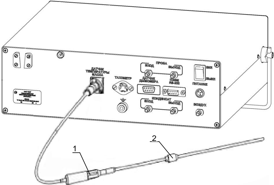
1 - Датчик температуры; 2 - Ограничитель Рисунок 8 - Подключение датчика температуры
