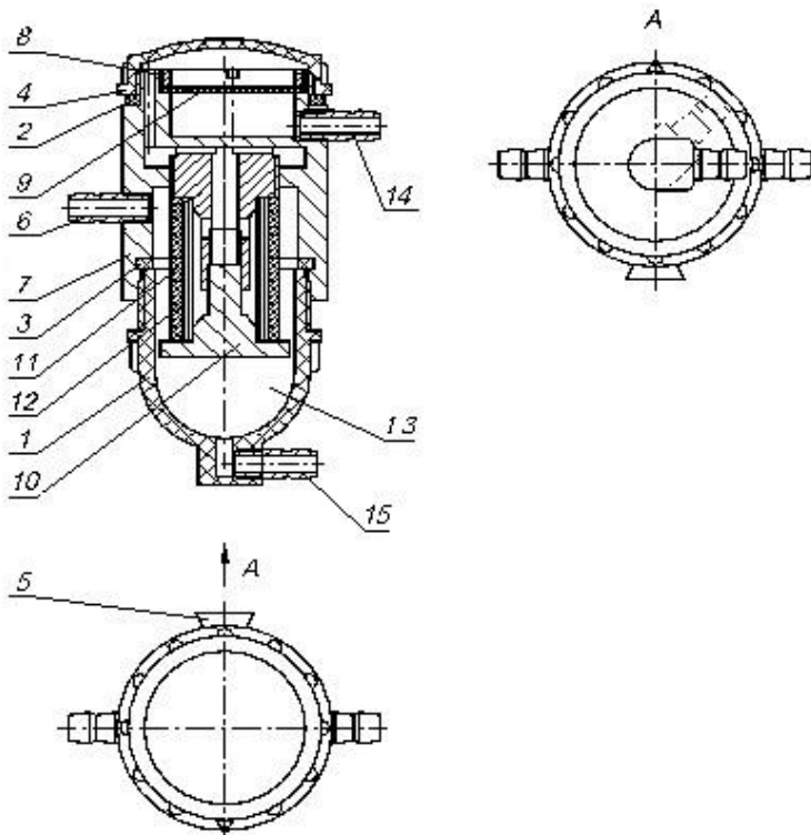
Рисунок 3 - Патрон фильтра грубой очистки
