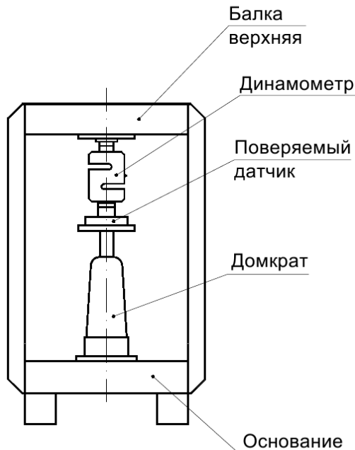
Рисунок 8. Силовозадающее устройство для проверки стэнда при измерении усилий вталкивания сцепного устройства
