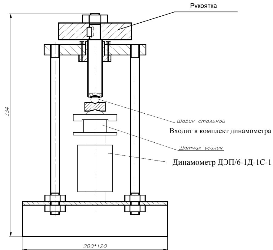
Рисунок 7 – Силозадающее устройство для проверки стенда при измерении усилия на органе управления
