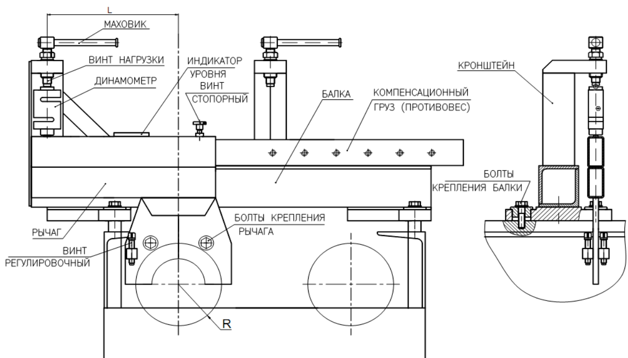
Рисунок 5 – Рычаг поверочный для проверки датчиков тормозной силы стенов
